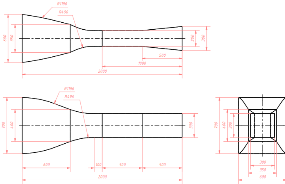
Gambar 3. Variasi desain 2
