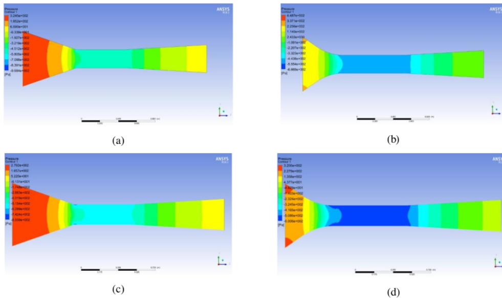
Gambar 11. Kontur tekanan udara wind tunnel : (a) Variasi model 1, (b) Variasi model 2, (c) Variasi model 3 dan (d) Variasi model 4
