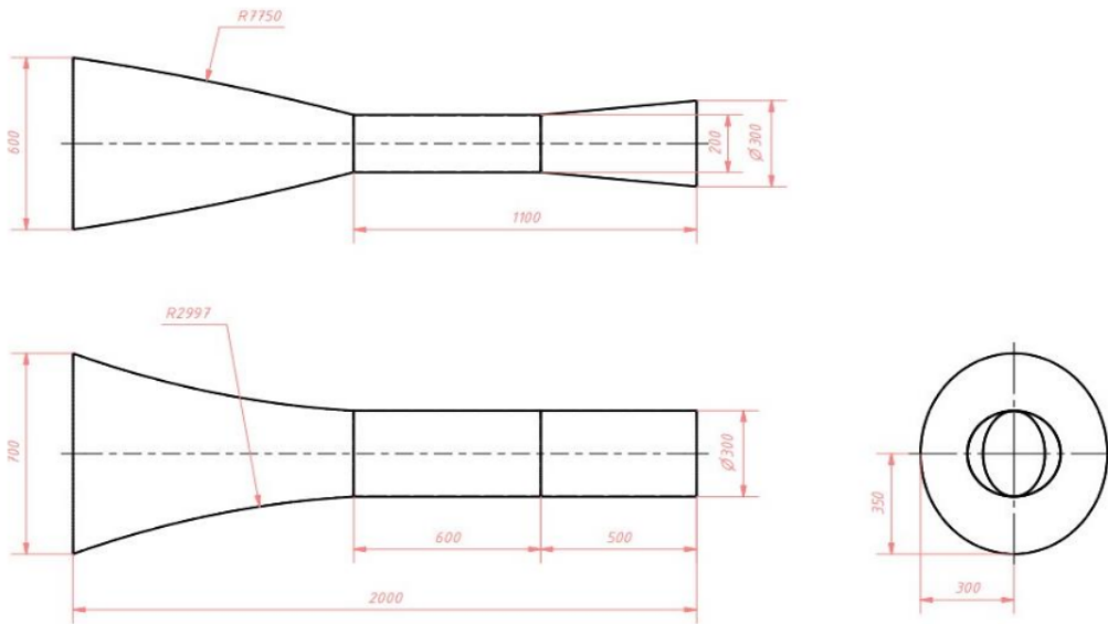
Gambar 5. Variasi desain 4
