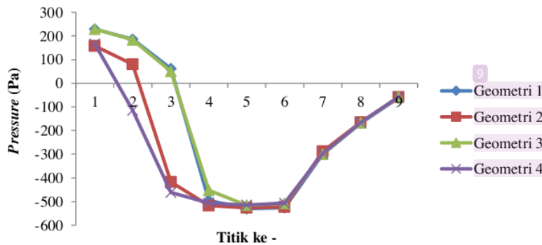
Gambar 12. Grafik tekanan udara di sembilan titik pengukuran
