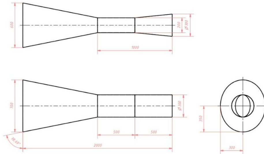
Gambar 4. Variasi desain 3
