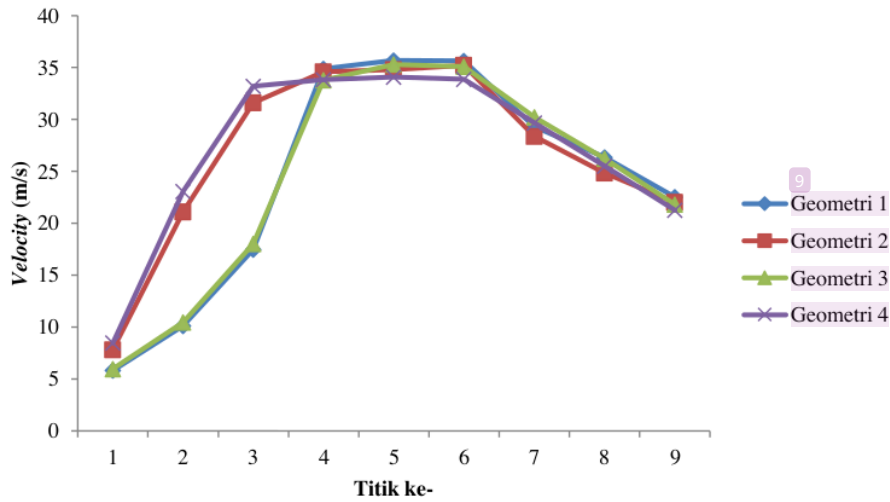
Gambar 10. Grafik kecepatan udara di sembilan titik pengukuran
