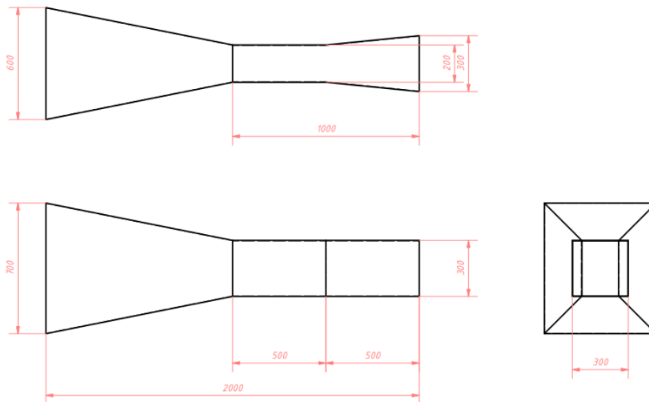
Gambar 2. Variasi desain 1
