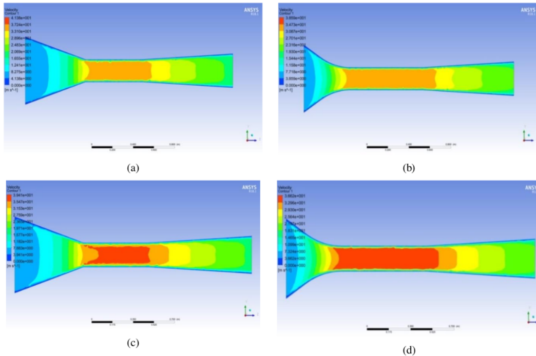
Gambar 9. Kontur kecepatan wind tunnel : (a) Variasi model 1, (b) Variasi model 2, (c) Variasi model 3 dan (d) Variasi model 4
