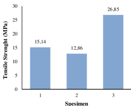
Gambar 4. Perbandingan nilai tensile strenght spesimen uji
