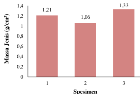
Gambar 2. Perbandingan nilai massa jenis spesimen uji
