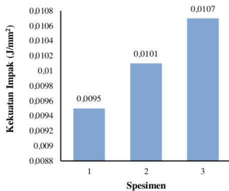
Gambar 3. Perbandingan nilai harga impact spesimen uji
