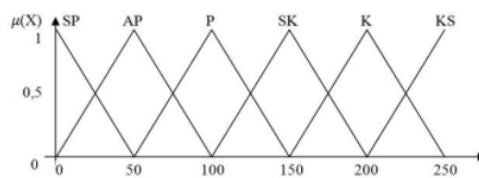
Gambar 5 Fuzifikasi Output Kipas
