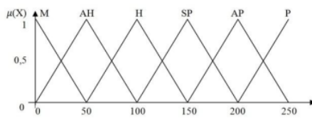
Gambar 4 Fuzzifikasi Output Heater
