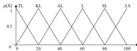
Gambar 3 Fuzzifikasi Input Kelembaban
