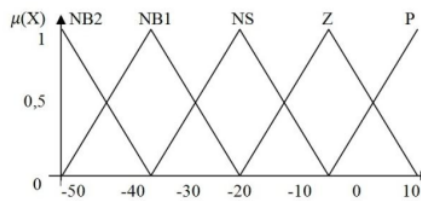
Gambar 2 Fuzzifikasi Input Error Suhu
