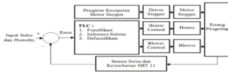
Gambar 1 Diagram Blok Sistem Pengeringan
