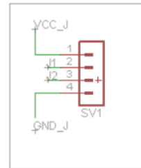
Gambar 4. Rangkaian Sensor HC-SR04
