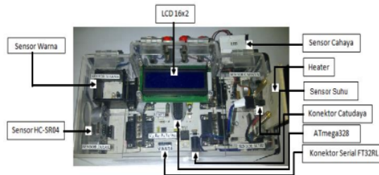
Gambar 8. Trainer Sensor Berbasis Arduino
