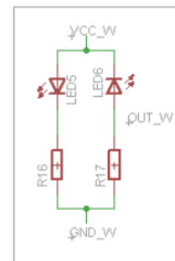
Gambar 6. Rangkaian Sensor Warna
