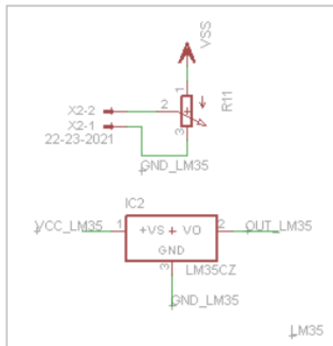
Gambar 3. Rangkaian Sensor LM35
