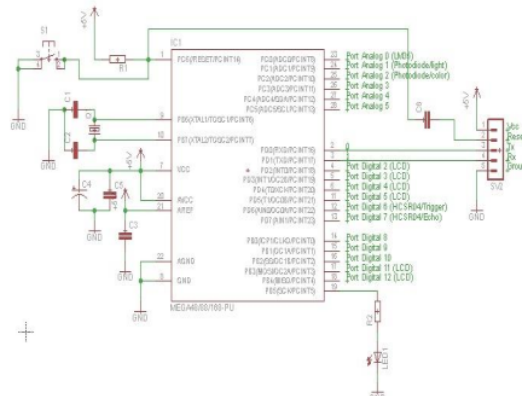
Gambar 1. Rangkaian mainboard
