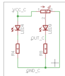
Gambar 5. Rangkaian Sensor Cahaya
