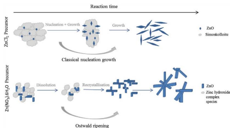
Gambar 5.3 . Pertumbuhan kristal ZnO dengan prekursor ZnCl 2 dan Zn(NO 3 ) 2 yang berbeda Ozel et al. , (2016)
