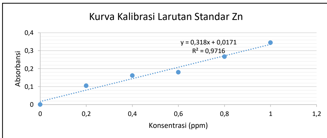
Gambar 5.10. Kurva kalibrasi larutan standar logam Zn
