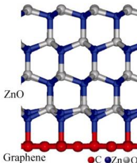
Gambar 2.5. Struktur kimia graphene-ZnO (Choi et al. , 2011)
