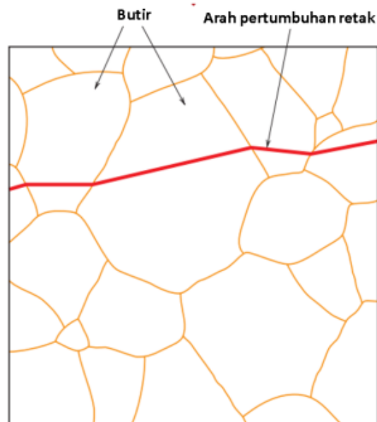
Gambar 8.21. Skema Terjadinya Transgranular Fracture
