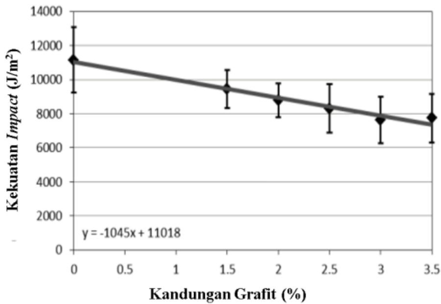
Gambar 8.16. Pengaruh Komposisi Grafit sebagai Aditif Terhadap Kekuatan Impact (Ando, 2018)
