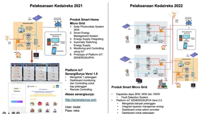
Gambar 1. Desain Platform IoT Senergisurya Smart micro Grid pada jaringan PLTS
