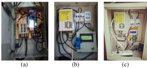
Fig. 2. IoT and Monitoring Module. a) IoT Module, b) Data Looger AC Module, c) Data Logger DC Module
