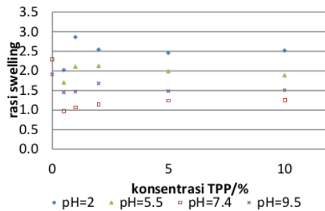
Gambar 6. Rasio swelling kitosan-tripolifosfat
