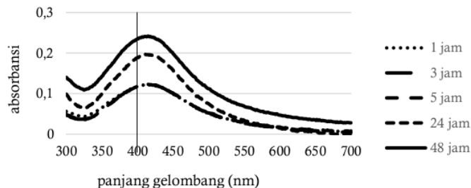
Gambar 3. Spektra UV-Vis yang menunjukkan hasil sintesis sampel B1 dengan penambahan PVA dan ekstrak secara selang-seling
