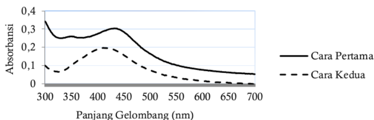
Gambar 2. Spektra UV-Vis yang menunjukkan perbandingan puncak serapan pada penambahan PVA dan ekstrak
