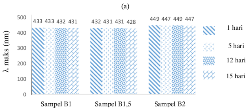
Gambar 6. Diagram yang Menunjukkan Pengaruh Volume Ekstrak terhadap (a) Nilai Absorbansi Maksimum, (b) Panjang Gelombang Maksimum Tiap Penambahan Waktu pada Sampel B ( \text{AgNO}_3 0,1 mM).
