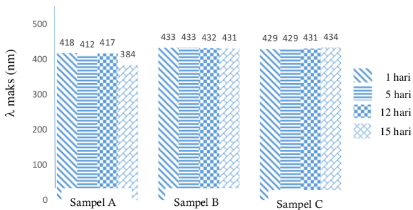
Gambar 5. Diagram pengaruh konsentrasi \text{AgNO}_3 terhadap perubahan panjang gelombang maksimum NPP. sampel A ( \text{AgNO}_3 0,05 mM), sampel B ( \text{AgNO}_3 0,1 mM), sampel C ( \text{AgNO}_3 0,25 mM).
