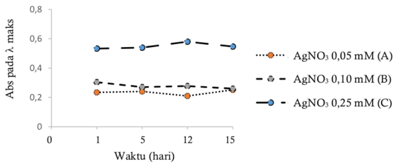
Gambar 4. Grafik yang menunjukkan pengaruh konsentrasi \text{AgNO}_3 terhadap absorbansi NPP selama 15 hari
