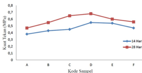
Gambar 2. Grafik hubungan komposisi agregat dengan kuat tekan pada batako umur 14 dan 28 hari
