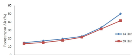
Gambar 1. Grafik hubungan komposisi agregat dengan penyerapan air pada batako umur 14 dan 28 hari
