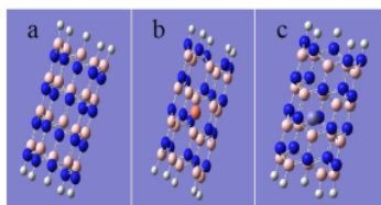
Gambar 1. struktur teroptimasi untuk: (a) BNNT, (b) BNNT disisipi logam Fe, (c) BNNT disisipi logam Cu
