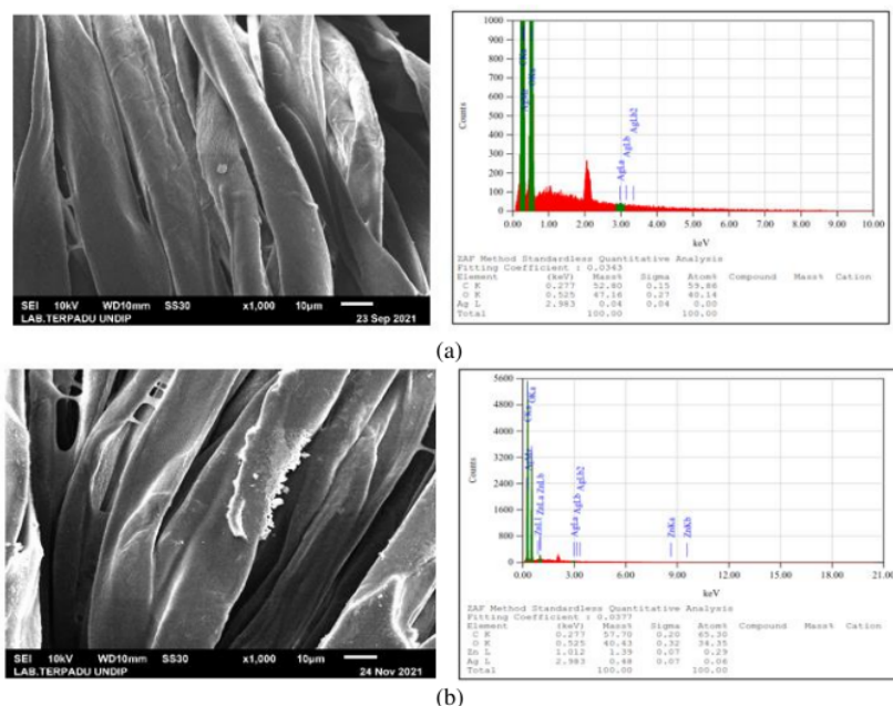
Gambar 7. Foto SEM dan data EDX kain terlapi NPP a) dengan 1x pencelupan dan b) dengan 3x pencelupan. Perbesaran foto SEM adalah 1000x, skala bar 10 \mu\text{m} .
