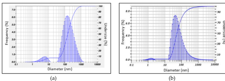
Gambar 2. Distribusi ukuran nanopartikel perak hasil sintesis dengan a) pemanasan konvensional dan b) irradiasi gelombang mikro
