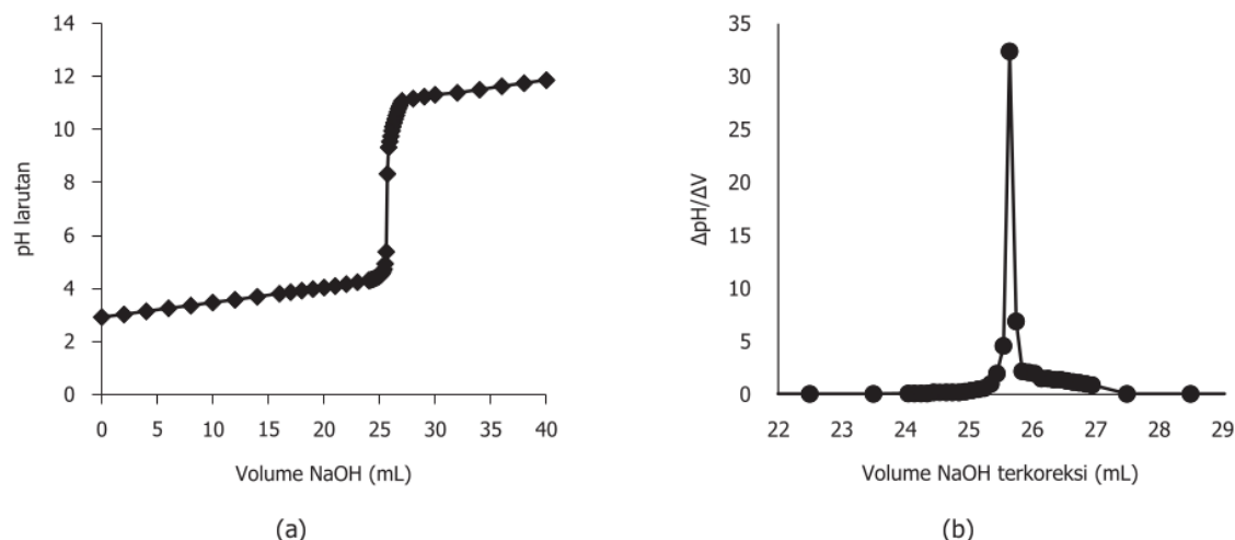
Gambar 3. Kurva titrasi \text{CH}_3\text{COOH} dengan \text{NaOH} (a) hubungan antara pH dengan volume titran, (b) kurva turunan pertama
