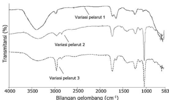
Gambar 1. Spektrum inframerah ekstrak pekat kulit buah naga dari 3 variasi pelarut
