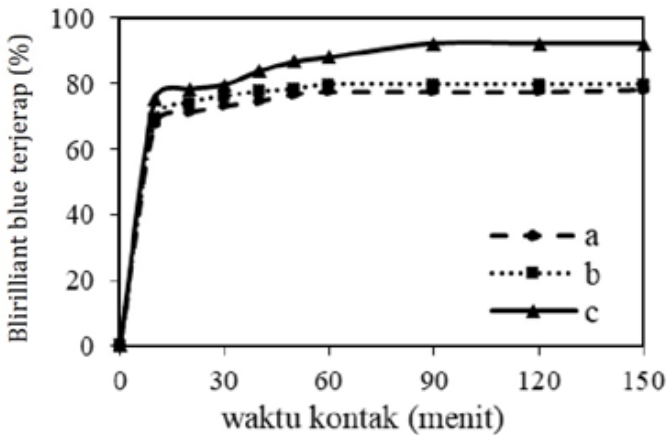
Gambar 6.12. Pengaruh waktu kontak terhadap persentase brilliant blue terjerap (a = Karbon Tanpa Aktivasi, b = CAC, c = MAC)
