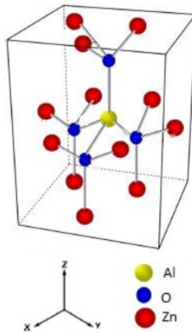
3 Gambar 7.2. Struktur Kristal ZnO:Al (Maldonado & Stashans, 2010)
