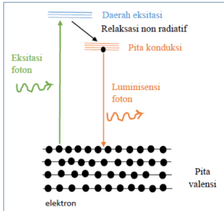
Gambar 7.4. Prinsip Spektroskopi PL
