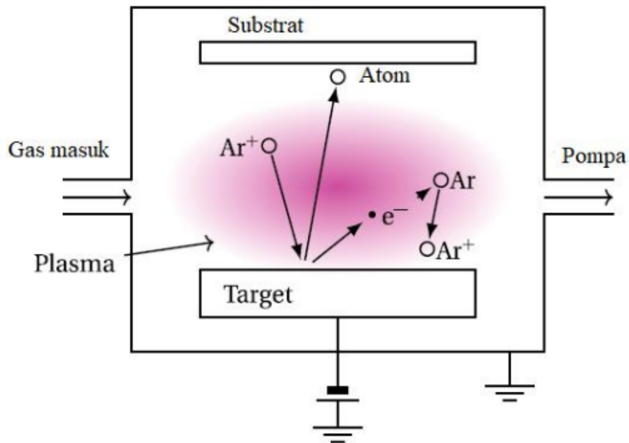
Gambar 7.11. Skematik Plasma Argon pada Sputtering (Mickan, 2017)
