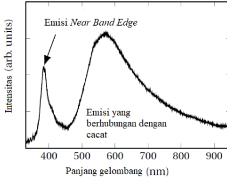
Gambar 7.5. Spektrum PL Film Tipis ZnO (Mickan, 2017)
