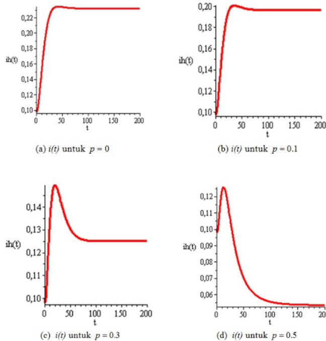
Gambar 3. Proporsi individu infectious untuk p = 0 , p = 0.1 , p = 0.3 , dan p = 0.5 .
