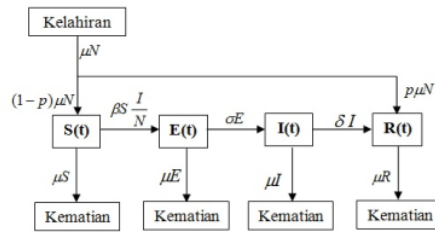
Gambar 1. Diagram Transfer Penyebaran Penyakit Campak dengan Pengaruh Vaksinasi
