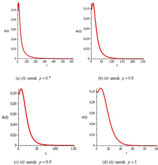
Gambar 4. Proporsi individu infectious untuk p = 0.7, p = 0.8, p = 0.9 , dan p = 1 .
