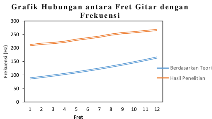
Gambar 2. Grafik Hubungan antara Fret Gitar terhadap Frekuensi
