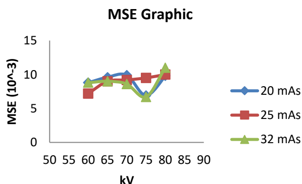
Gambar 2. Grafik hubungan antara tegangan tabung sinar X dengan nilai MSE citra
