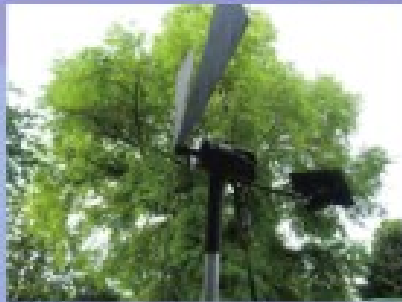
MODEL PEMBANGKIT LISTRIK TENAGA ANGIN DAN SURYA SKALA KECIL UNTUK DAERAH PERBUKITAN
