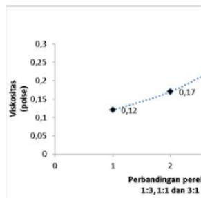
Gambar 3. Hubungan antara perbandingan bobot tepung tapioka dengan kapur tohor terhadap viskositas cat.
