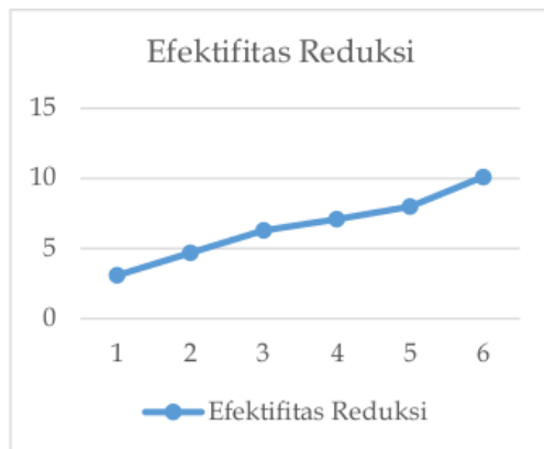
Gambar 3. Grafik Hubungan Komposisi Ampas Teh dengan Angka Efektivitas Reduksi Kebisingan yang Dihasilkan
