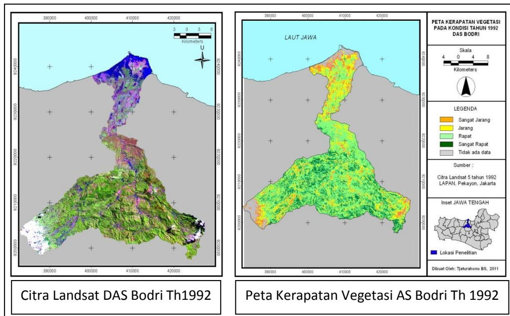
Gambar 2. Citra landsat 5 Tahun 1992 dan Peta Kerapatan Vegetasi DAS Bodri
