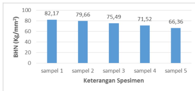
GAMBAR 4. Grafik Nilai Kekerasan Brinell pada Bahan Komposit Kampas Rem
