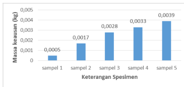
GAMBAR 5. Grafik Massa Keausan pada Bahan Komposit Kanvas Rem
