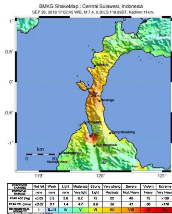
圖六 2018.9.28 M_w 7.5 Palu-Donggala 地震等震度圖 (PuSGeN, 2018)
