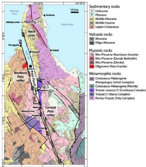
(a) Palu 地區地質環境背景-基岩分佈 (Watkinson, 2011; GEER, 2019)
