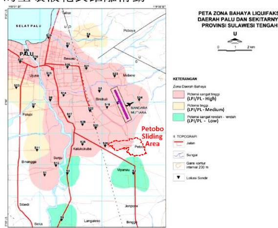
圖五 Palu 地區前期土壤液化潛能分析 (Widyaningrum, 2012; PuSGeN, 2018)
