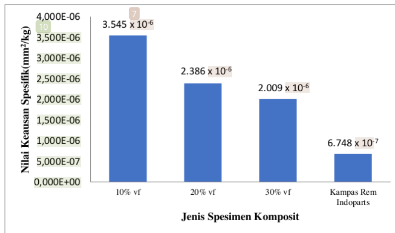
Gambar 2. Grafik Nilai Keausan Spesifik
