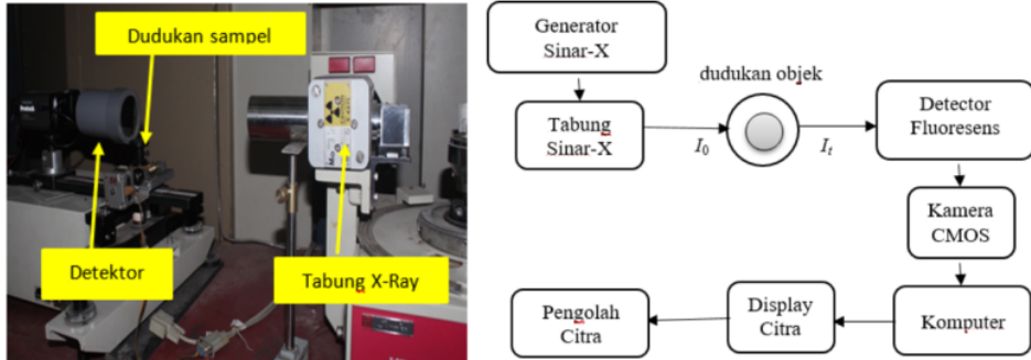
Gambar 3: Susunan instrumen dan skema mikro-radiografi sinar-X digital.
