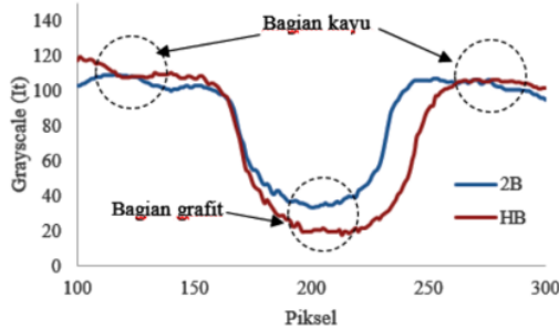
Gambar 7: Grafik profil intensitas transmisi sinar-X pada citra pensil untuk bagian kayu dan grafit.
