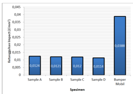
Gambar 6. Grafik rata-rata ketangguhan impact spesimen
