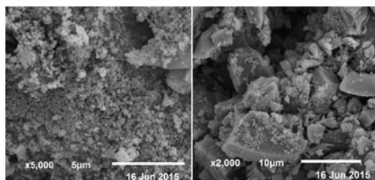
Fig. 3. SEM images for nanosized TiO 2 -SiO 2
