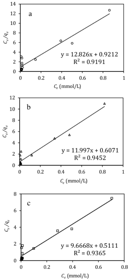
Gambar 7. Model kesetimbangan Langmuir pada adsorpsi methyl violet oleh karbon teraktivasi ZnCl_2 dengan konsentrasi (a) 10%, (b) 20%, dan (c) 30% dan pemanasan gelombang mikro
