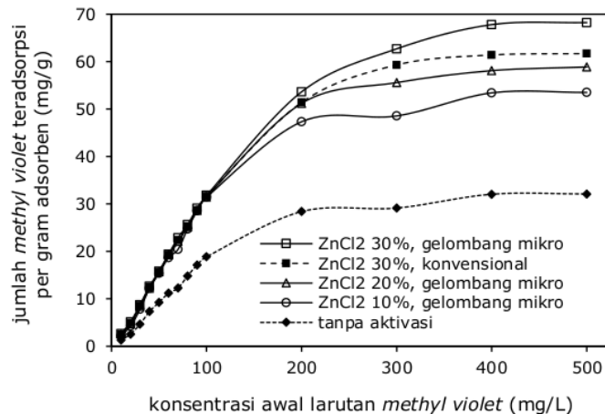
2 Gambar 4. Pengaruh konsentrasi awal larutan terhadap jumlah methyl violet teradsorpsi (kondisi proses: pH 3, waktu kontak 180 menit, dosis karbon aktif 0,3 gram/50 mL larutan)
