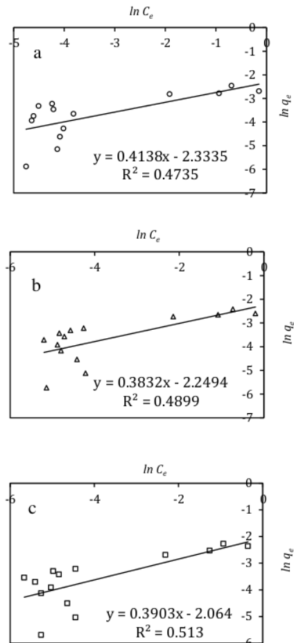
Gambar 8. Model kesetimbangan Freundlich pada adsorpsi methyl violet oleh karbon teraktivasi ZnCl_2 dengan konsentrasi (a) 10%, (b) 20%, (c) 30% dengan pemanasan gelombang mikro
