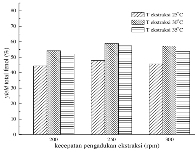
Gambar 4. Hubungan antara Yield Total Fenol Hasil Ekstraksi Bio-oil pada Suhu Pirolisis Bagas Tebu 500°C dengan Kecepatan Pengadukan dan Suhu Ekstraksi
