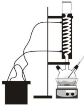
Gambar 1. Rangkaian Alat Ekstraksi Fenol dari Bio-Oil
