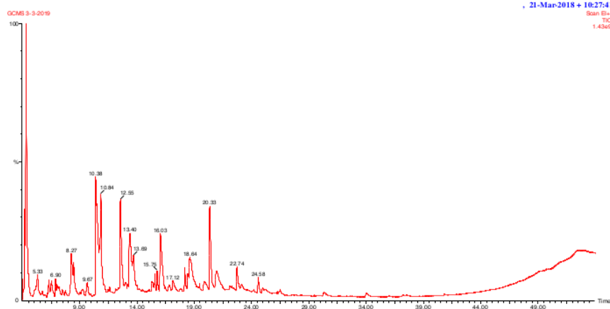
Gambar 2. Kromatogram Bio-Oil Hasil Pirolisis Bagas Tebu Suhu 500°C
