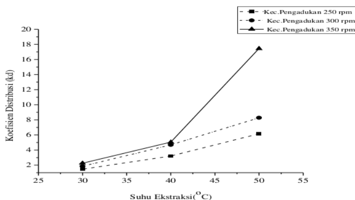
Gambar 6. Pengaruh Suhu dan Kecepatan Pengaduka Terhadap Koefisien Distribusi pada Ekstraksi Fenol
