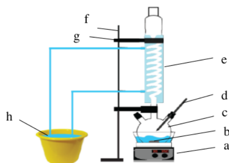
Gambar 2. Rangkaian Alat Ekstraksi
