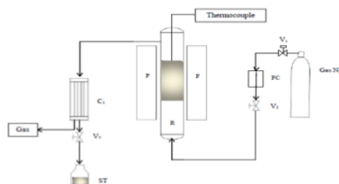
Gambar 1. Rangkaian Alat Pirolisis
