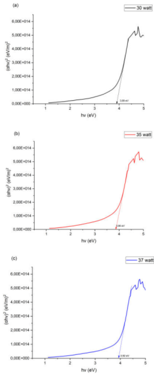
1 Gambar 4.5 Band gap film tipis ZnO:Ga yang ditumbuhkan dengan variasi daya plasma
