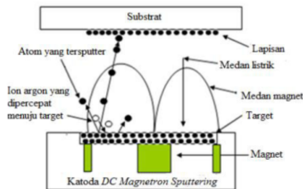
Gambar 3.1 Skema reaksi dalam DC magnetron sputtering (Joshi, 2003)
