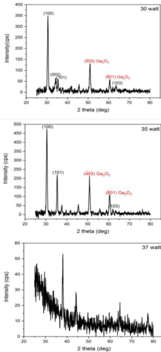
3 Gambar 4.1 Spektrum XRD film tipis ZnO:Ga dengan variasi daya plasma
