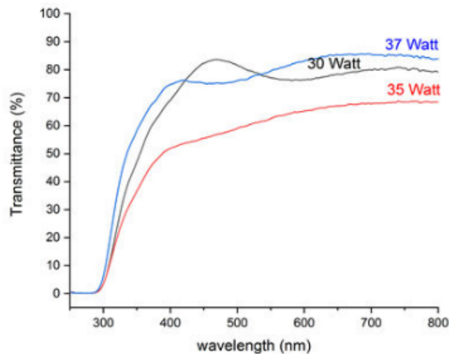
3 Gambar 4.4 Grafik transmittansi film tipis ZnO:Ga variasi daya plasma
