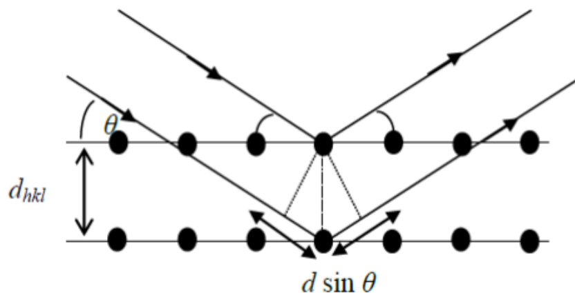
Gambar 3.3 Hamburan sinar-X pada kristal
