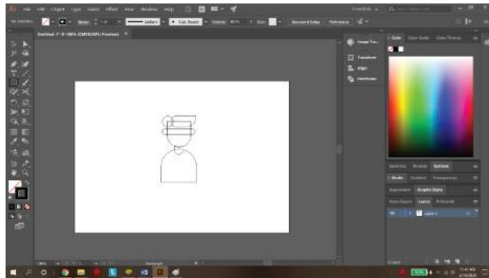
Gambar 3.6 Menggambar objek
