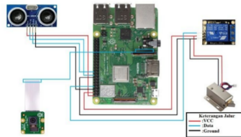
Gambar 1. Diagram blok pengenalan wajah menggunakan Raspberry Pi
