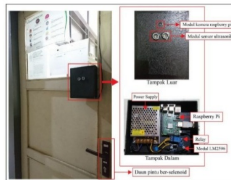
Gambar 5. Setup dan aplikasi keamanan pintu rumah pintar menggunakan pengenalan wajah
