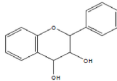
Gambar 2. Struktur Inti Tanin (Harborne, 1987 dalam Ummah, 2010:18)
