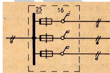
Gambar 3.a. Diagram rangkaian Gambar 3.b. Bentuk kontak hubung bagi
